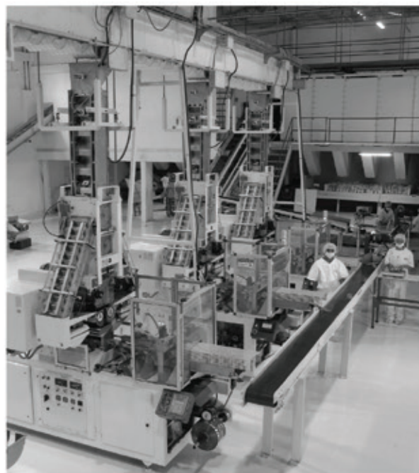
Línea de empaque de pasta larga
